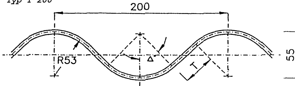
Typ T 200
